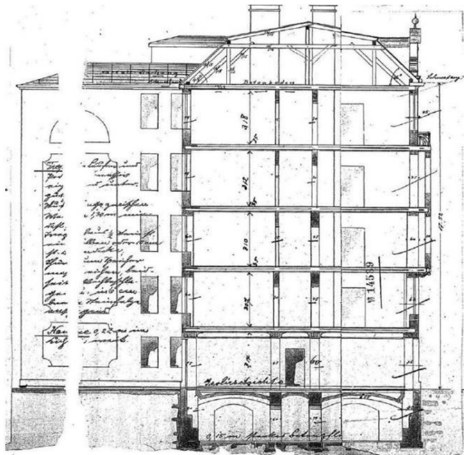
Schnitt Gebäude
