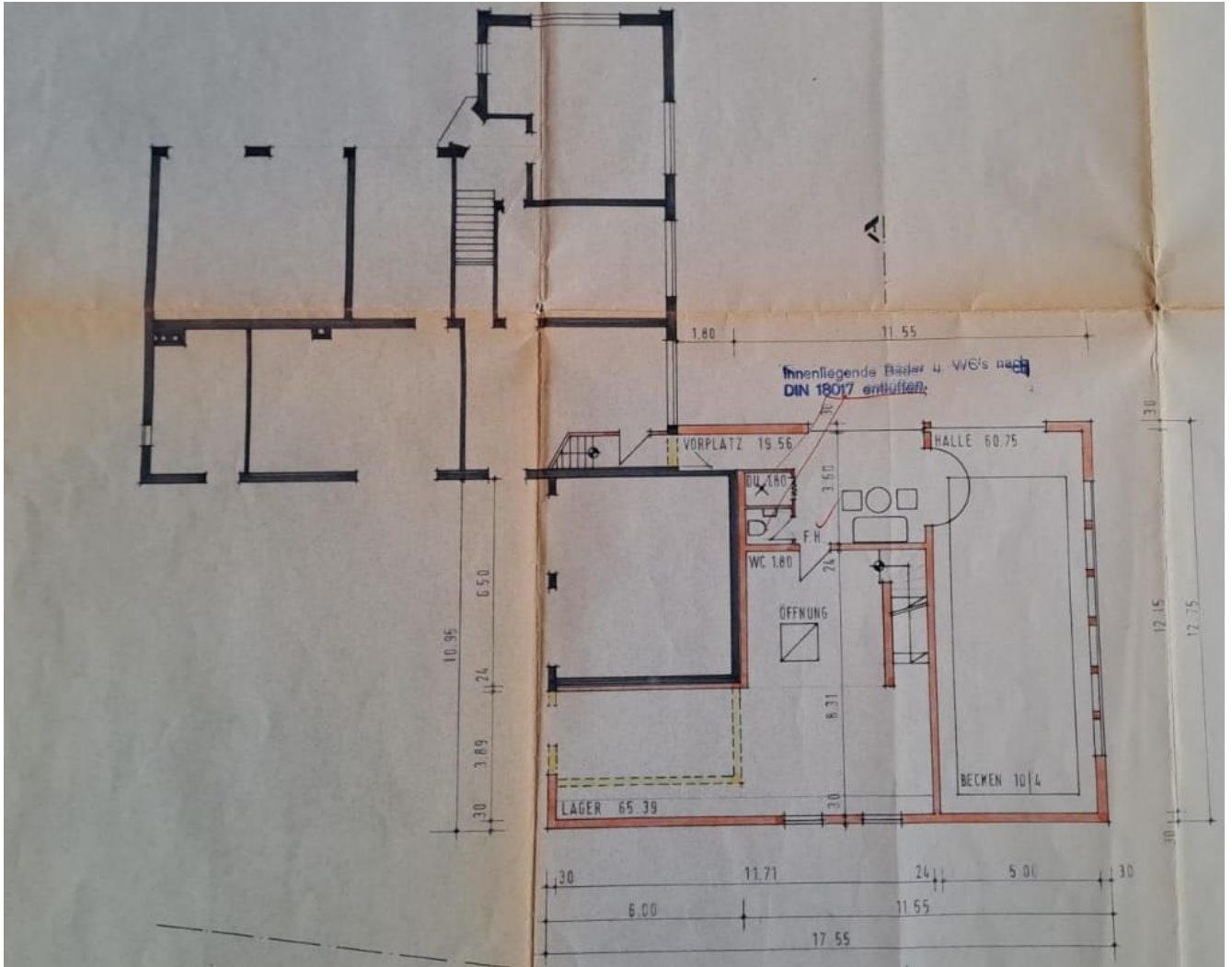
Grundriss Erdgeschoss
