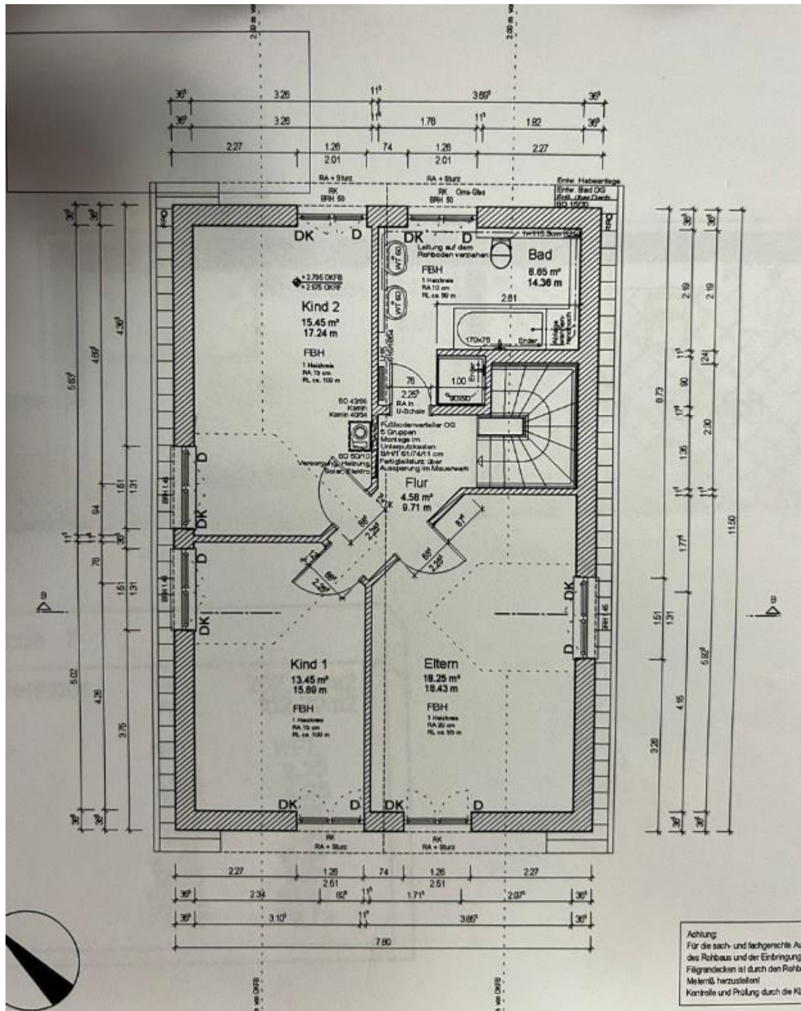
Grundriss DG
