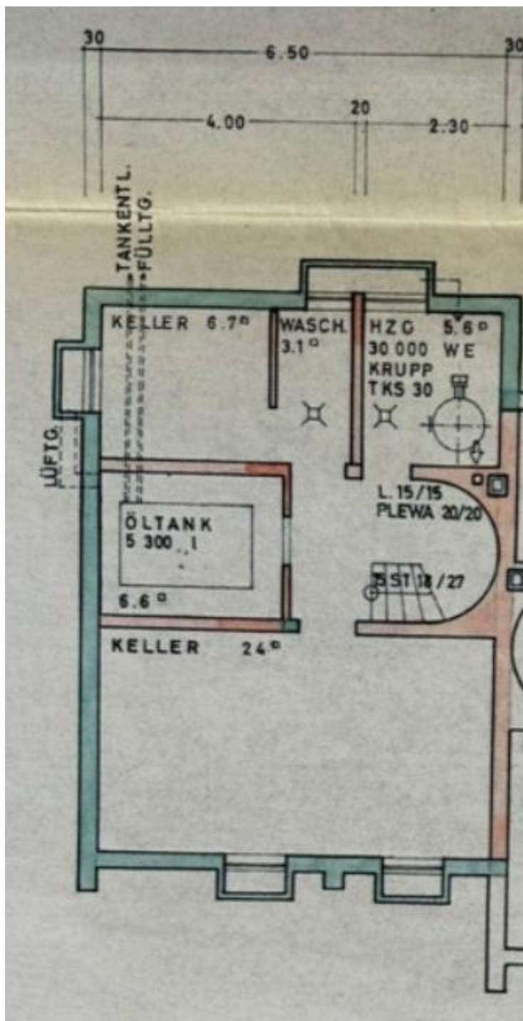
Grundriss KG
