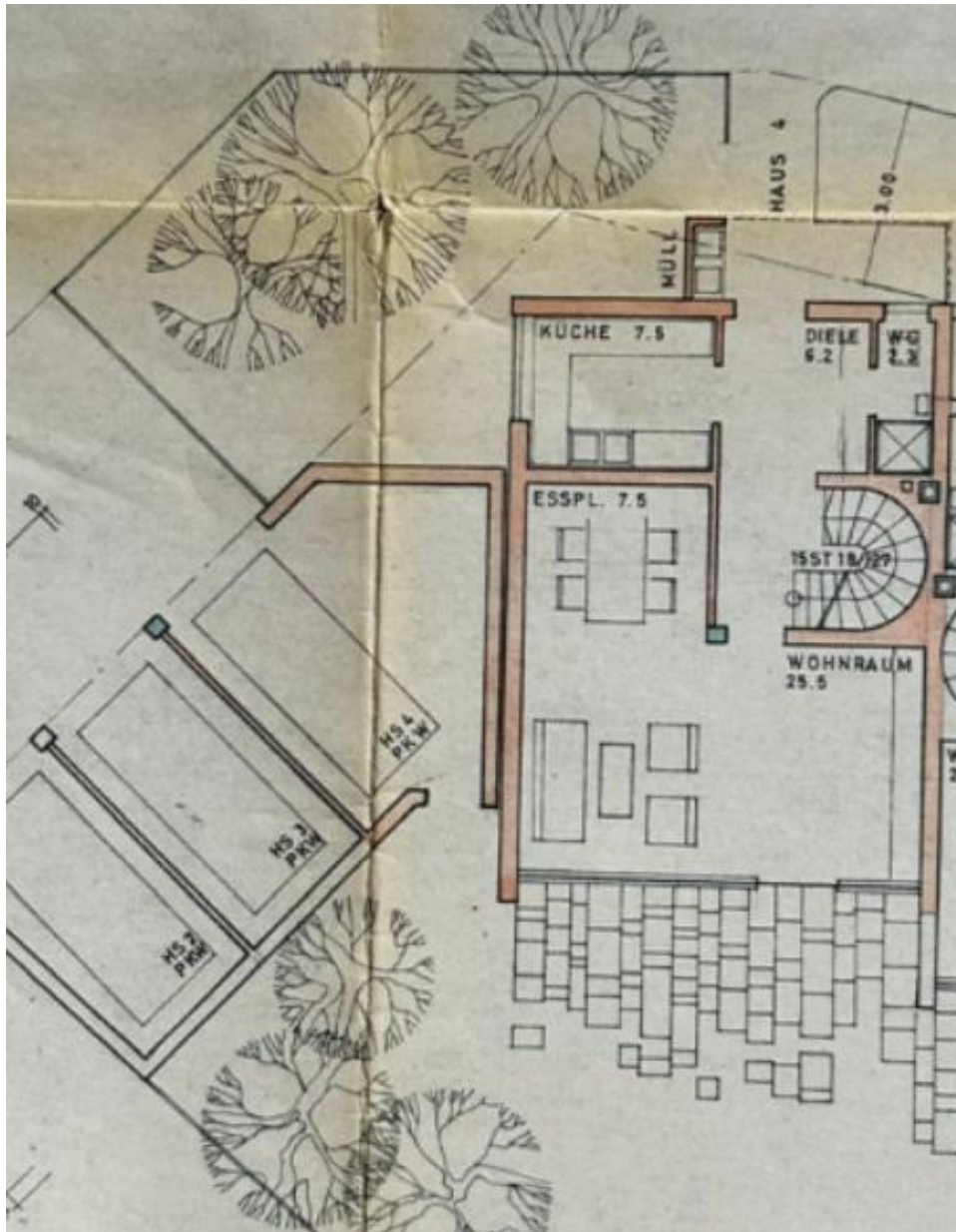
Grundriss EG
